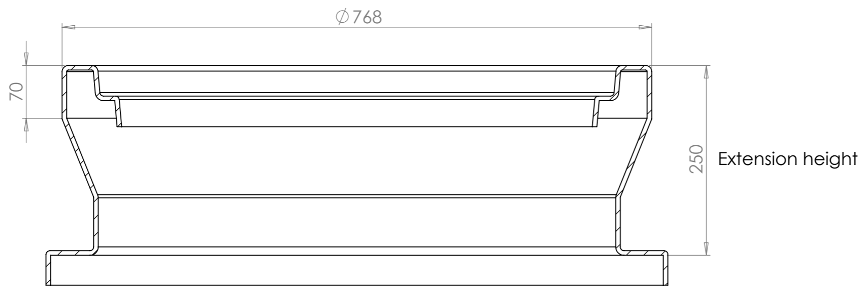
SECTION A-A SCALE 1 : 5
